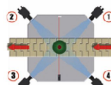
罐外壁检测原理图
